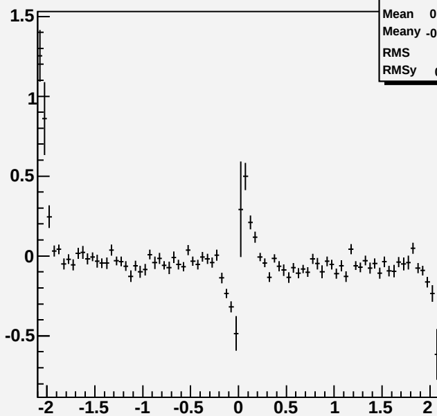
res_cell
