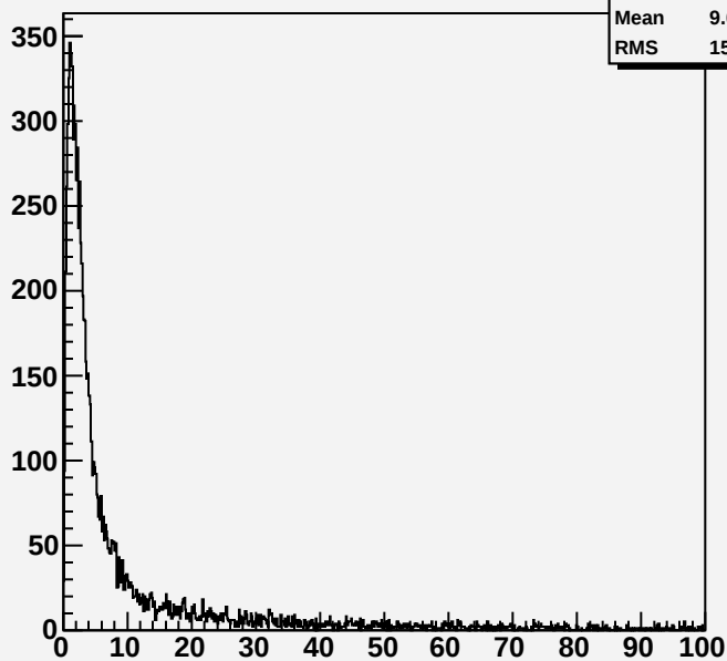
N / chi2min
