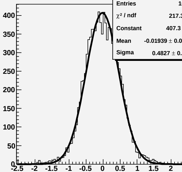
residuiold
