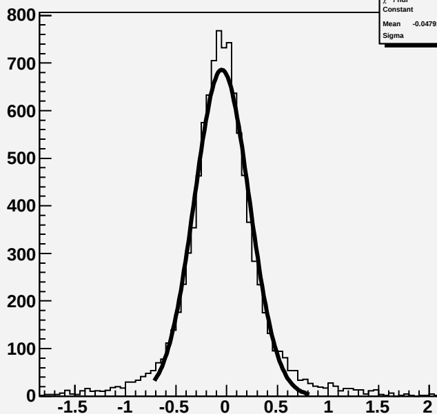
residuitest
