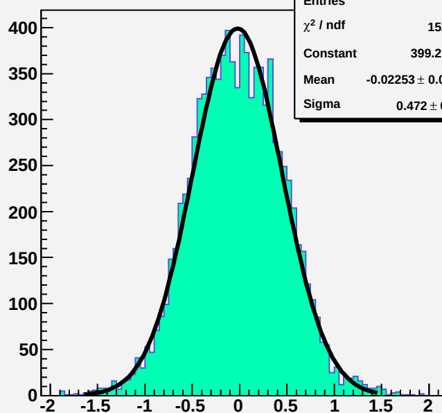
residuiold
