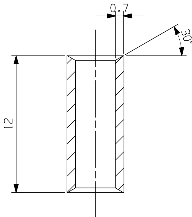
Sezione A-A
