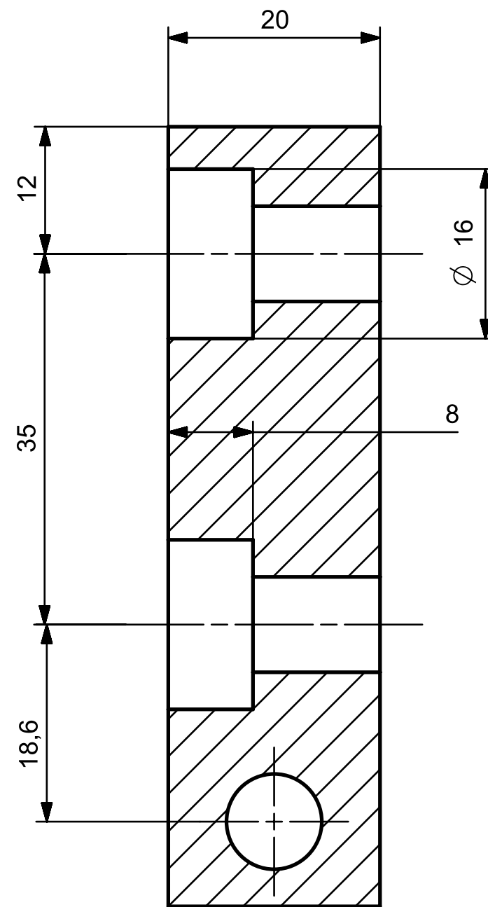
SECTION A-A
