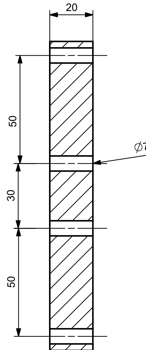
SECTION D-D
